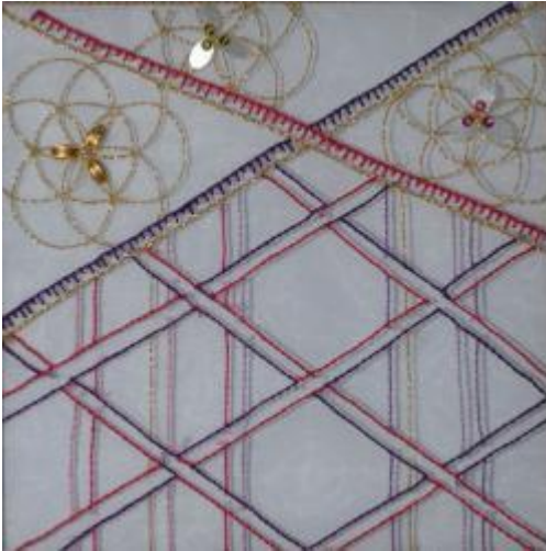
1-Origami
